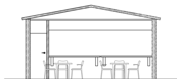
Prospetto laterale - scala 1:100
